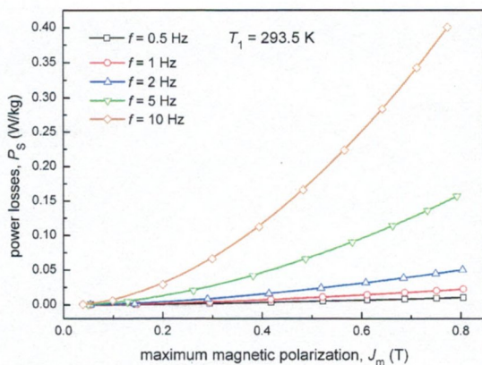
Rys. 1. Straty mocy dla stopu \text{LaFe}_{10.8}\text{Co}_{1.1}\text{Si}_{1.1} zmierzone w temperaturze T_1 = 293.5 \text{ K}
