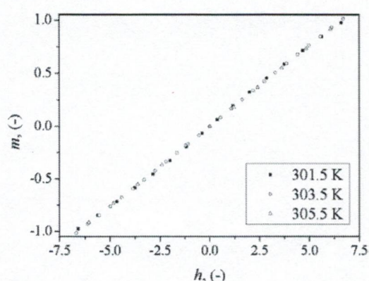
Rys. 2. Wyskalowane krzywe bezhistereowe dla temperatur powyżej przejścia fazowego
