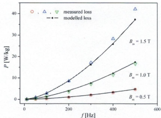
Rys. 3. Modelowanie krzywych stratności dla orientowanej blachy elektrotechnicznej
